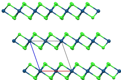
Krystalová struktura \alpha -IrCl 3 . 49
