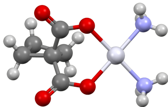
Kuličkový model karboplatiny. 38
