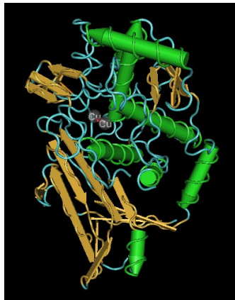
Molekulová struktura hemocyaninu. 39
