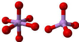
Koordinační polyedry v \text{As}_4\text{O}_{10} . 93
