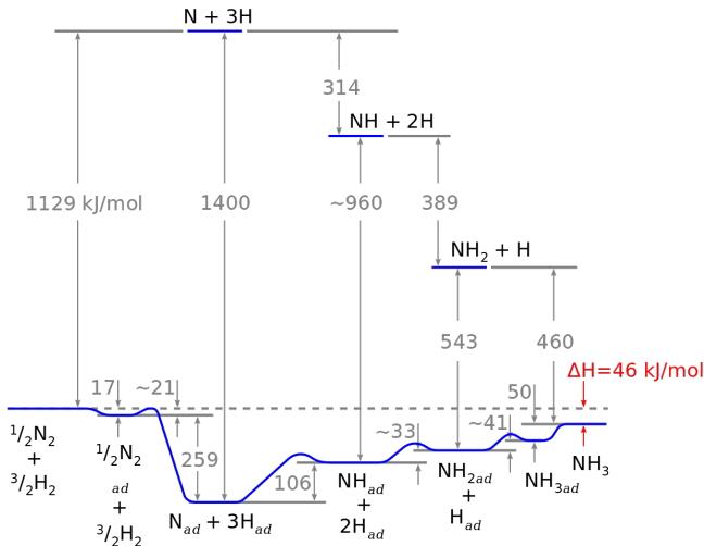
Energetický profil syntézy amoniaku. 3
