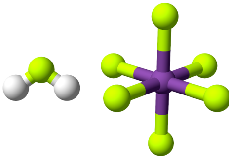
Model kyseliny hexafluoroantimoničné. 104
