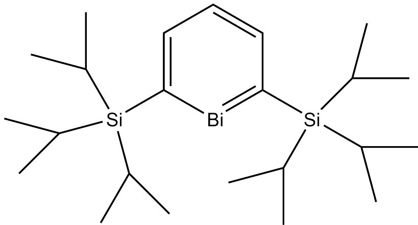
Stabilní derivát bismabenzenu 121
