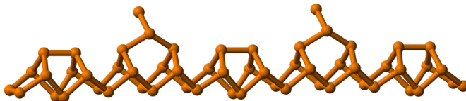
Krystalová struktura fialového fosforu. 7
