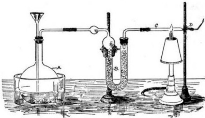
Aparatura na Marshovu zkoušku. 87
