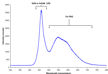
Spektrum bílé LED. 89
