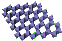
Krystalová struktura \text{FeCl}_3 . 115
