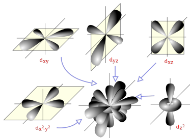
Tvary d-orbitalů. 41
