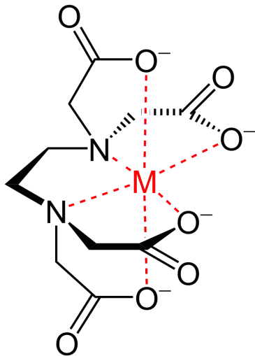
Iont kovu chelatovaný EDTA
