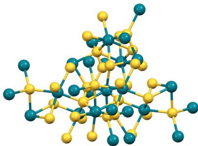
Struktura sulfidu rhoditého. 59
