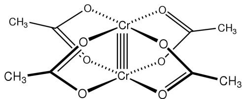
Octan chromnatý. 80
