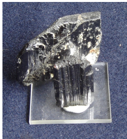
Wolframit. 52
