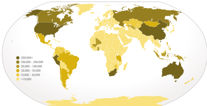
Mapa získávání zlata. 51
