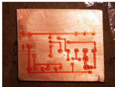
Cuprexitová destička pro přípravu DPS. 56
