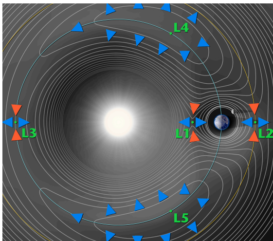
Lagrangeovy body Země. 82
