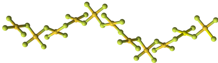
Krystalová struktura \text{AuF}_3 . 111
