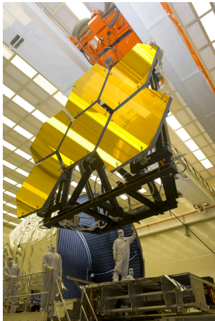
Zrcadlo JWST. 85
