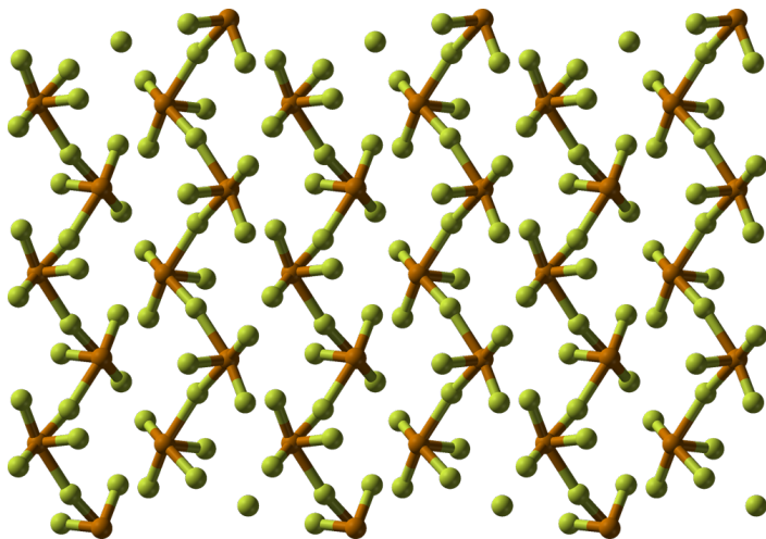
Krystalová struktura \text{TeF}_4 . 91
