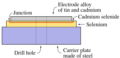
Struktura selenového usměrňovače. 59
