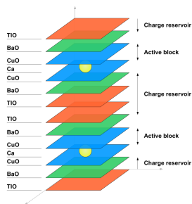
Struktura \text{TlBaCaCuO} . 48
