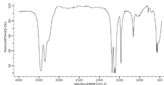
IR Absorption Spectrum
