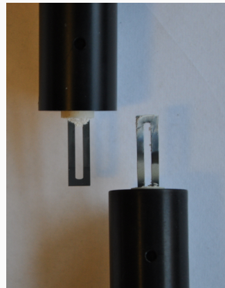
Nový a použitý globar
