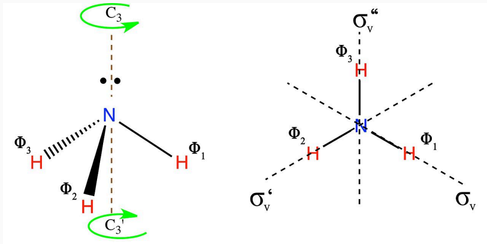
Operace symetrie v molekule amoniaku. 7
