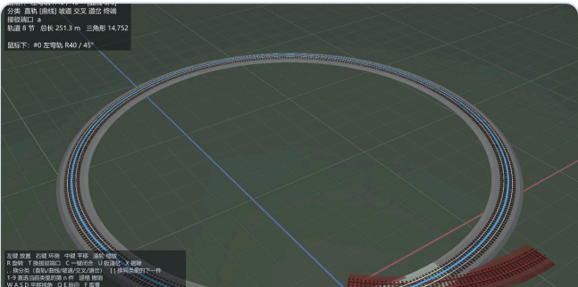
铺轨中 幽灵件吸附到最近的空闲端口，绿色即「可以放」
