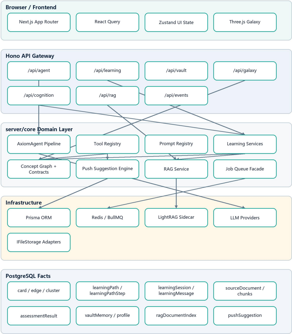
图 2 9. 技术架构图草案 (流程/架构图)
