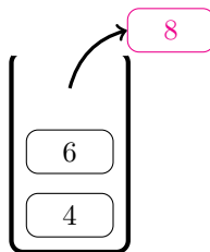
Pop
