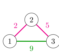
BFS
