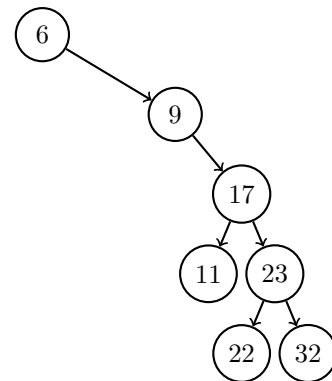
Splay 6 (zigzig)
