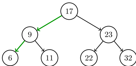
Insert 6
