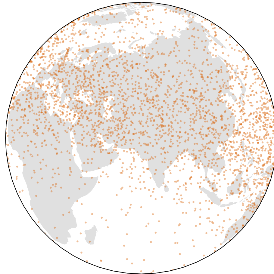
Malliavin
