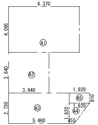
1階床面積図 S=1/200
