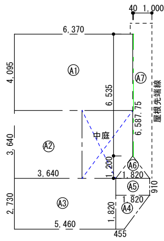
建築面積求積図 S=1/200
