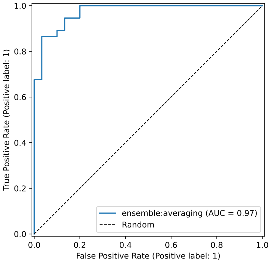
ROC Curve (AUC = 0.9730)
