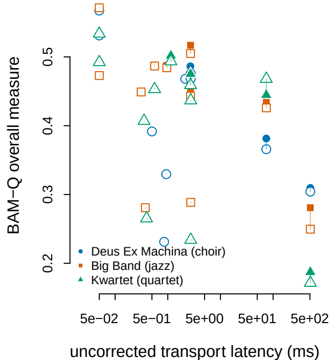
(b) BAM-Q
