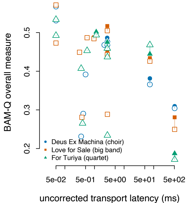
(b) BAM-Q
