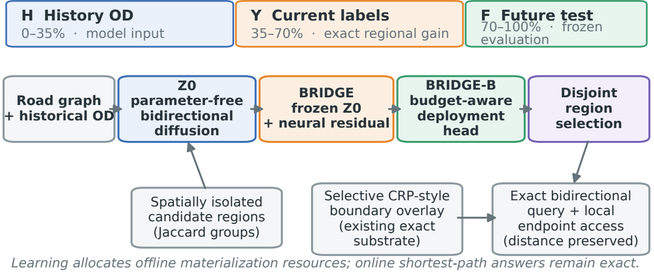
图 1: 本文端到端方法。底层覆盖图采用已有精确索引结构, 本文研究重点是历史起终点需求驱动的区域排序、隔离与选择性物化; 学习只负责离线资源配置, 在线查询始终保持精确。
