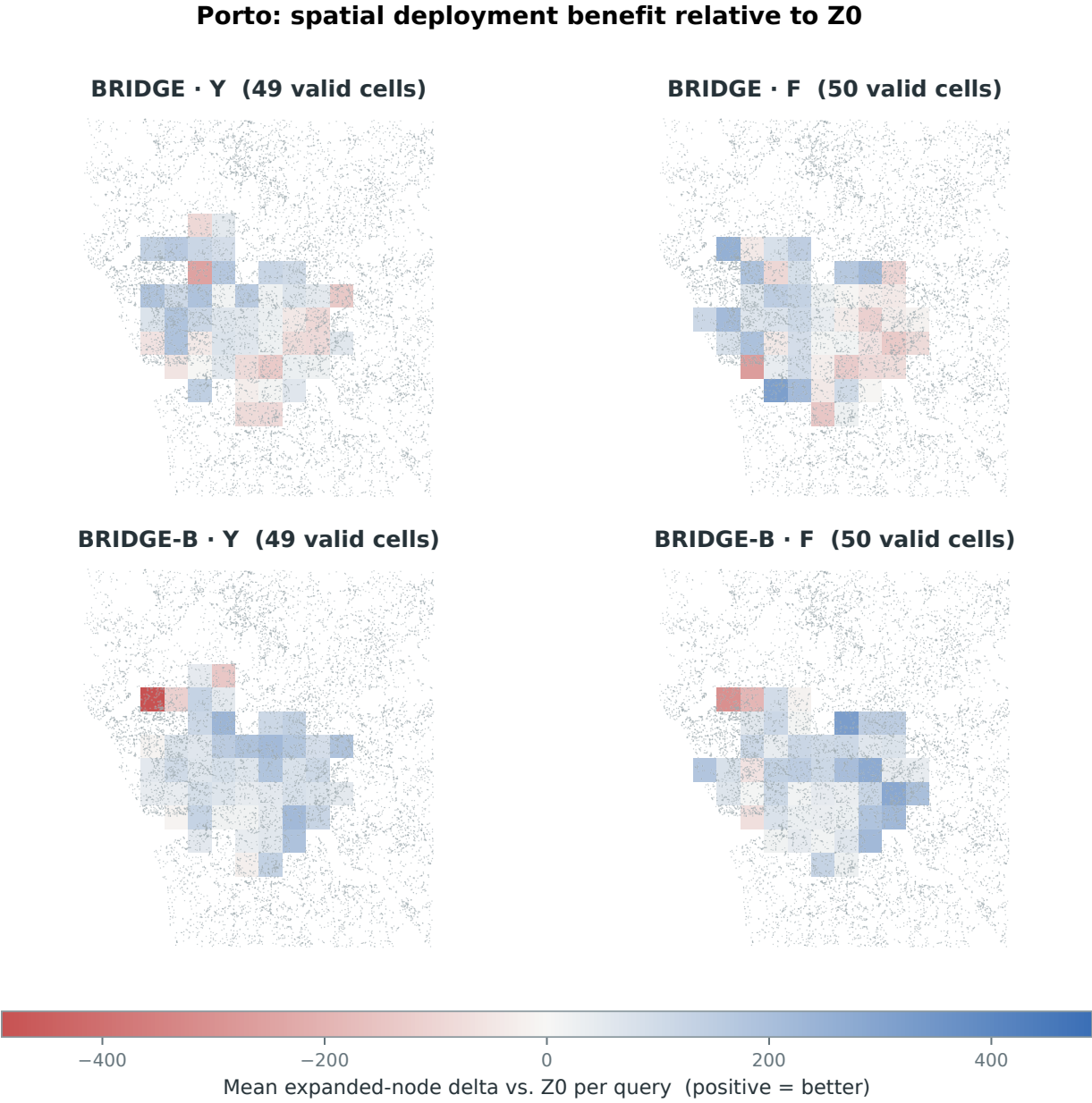
图 6: Porto 中 BRIDGE 与 BRIDGE-B 相对 Z0 的 Y/F 逐查询展开节点空间差。蓝色表示神经方法更少展开；BRIDGE-B 的正收益覆盖在两个窗口均较广。
