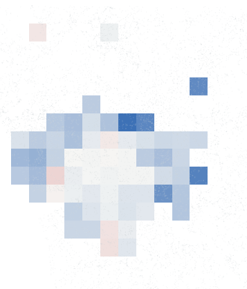
BRIDGE-B · F-D 63 valid cells
