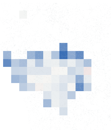
BRIDGE-B · Y-D 58 valid cells
