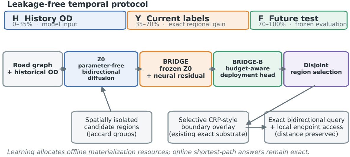
图 1: 本文端到端方法。底层覆盖图采用已有精确索引结构，本文研究重点是历史起终点需求驱动的区域排序、隔离与选择性物化；学习只负责离线资源配置，在线查询始终保持精确。
