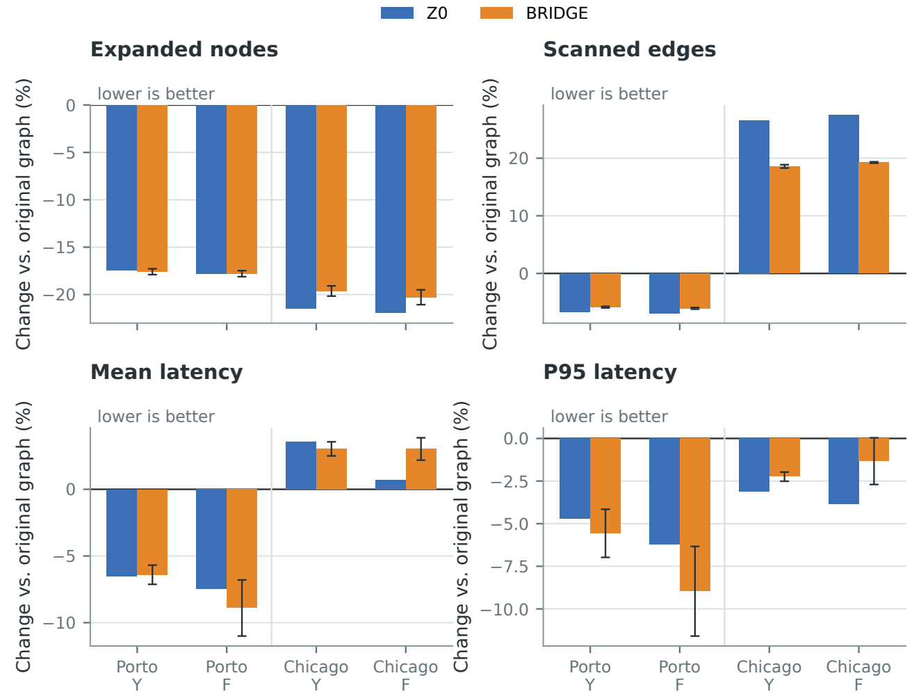
图 5: C++20/O3 同实现下, 选择性物化在两城中的系统收益与成本。负值表示相对原图减少; Chicago 虽减少展开节点, 却因密集 shortcut 增加扫边量, 说明排序收益与墙钟加速并不等价。
