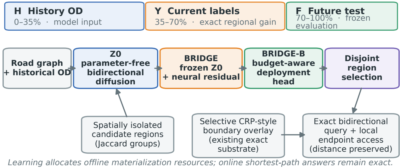
图 2: 本文端到端方法。底层覆盖图采用已有精确索引结构, 本文研究重点是历史起终点需求驱动的区域排序、隔离与选择性物化; 学习只负责离线资源配置, 在线查询始终保持精确。
