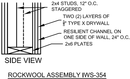
FIRE SEPARATION WALL #2A SCALE: 1" = 1'0" (11x17)
