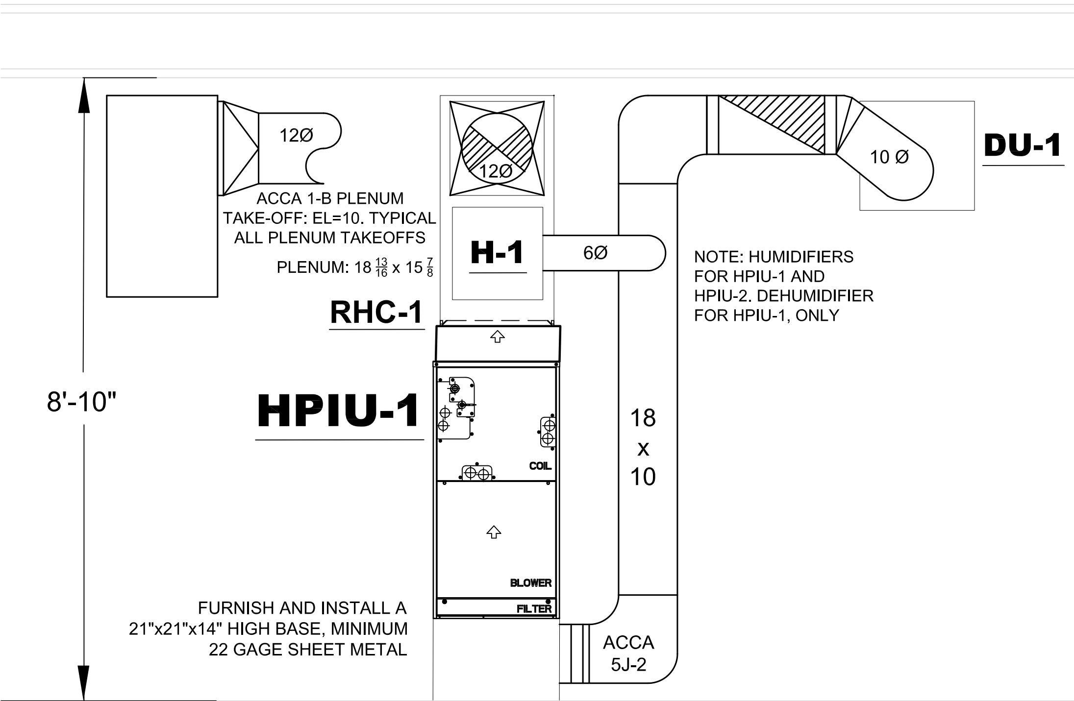
SECTION A-A SCALE: \frac{3}{4} = 1'0''
