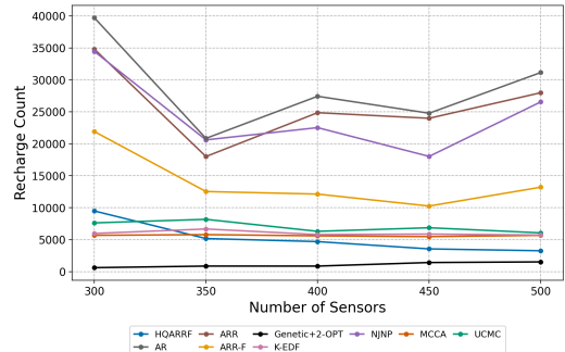
圖 13(b). 不同感測節點數量下各方法的基地台回充次數
