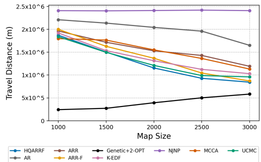
圖 9. 不同場域大小下各方法的總移動距離
