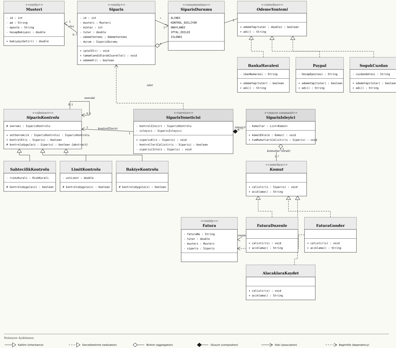
Şekil 2.1 · SimpleCar E-Satış — UML 2.x sınıf diyagramı. Sol kanat: CoR (kontroller); orta: orchestrator; sağ üst: Strategy (ödeme yöntemleri); sağ alt: Command (sıralı işleme adımları).
