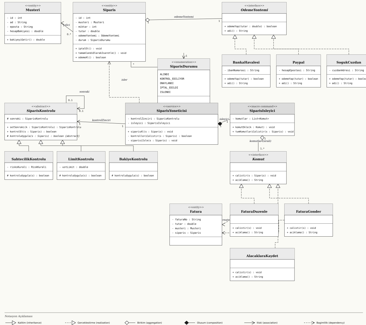
Şekil 2.1 · SimpleCar E-Satış — UML 2.x sınıf diyagramı. Sol kanat: CoR (kontroller); orta: orchestrator; sağ üst: Strategy (ödeme yöntemleri); sağ alt: Command (sıralı işleme adımları).
