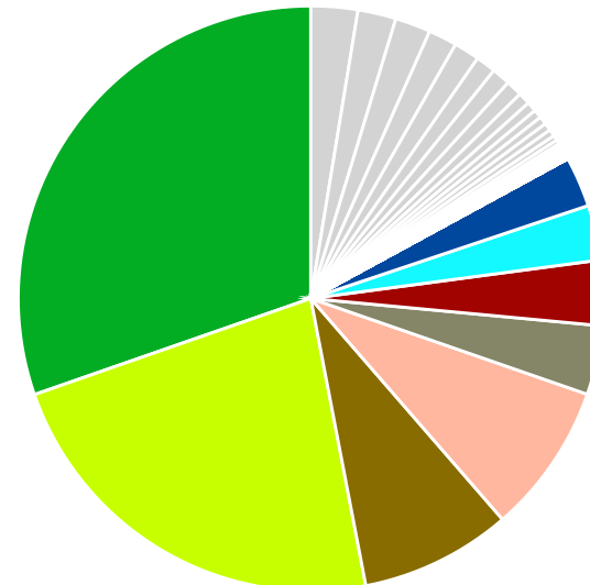
ME-16s
