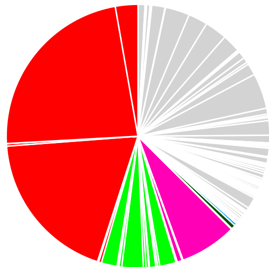
ME
