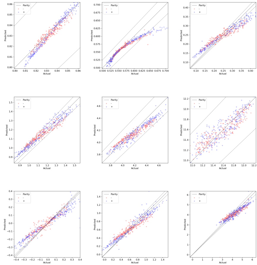
FIG. 3: Z
