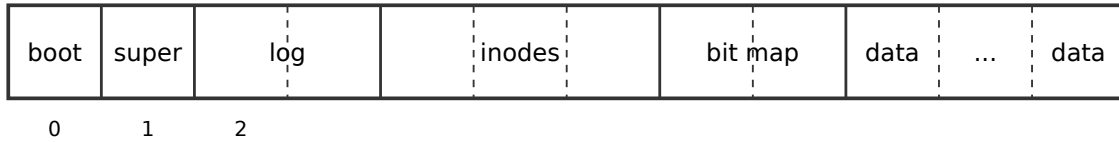
شكل 14: هيكلية تقسيم القرص بداخل نظام الملفات في xv6.
