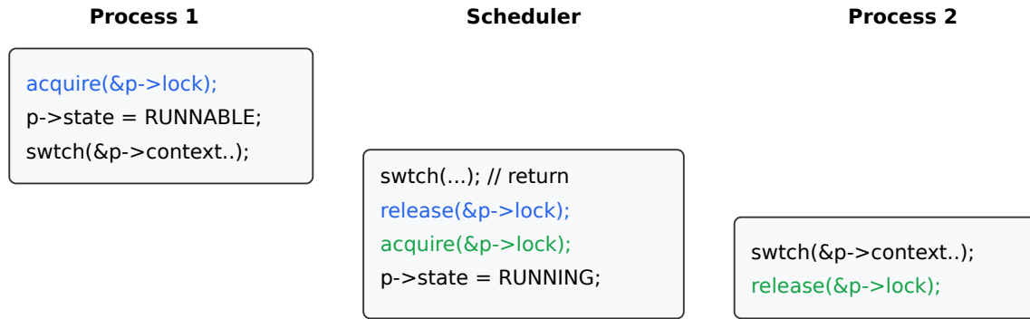
شكل 12: حيازة p-&gt;lock عبر الاستدعاءات لـ swtch.
