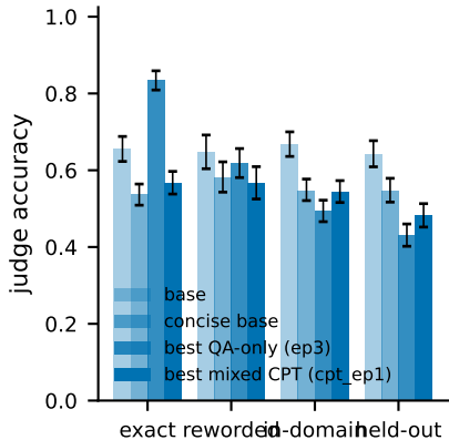
Qwen3-8B
