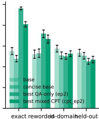
Llama 3.1 8B
