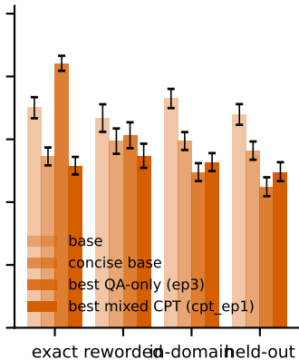
Gemma 4 E4B
