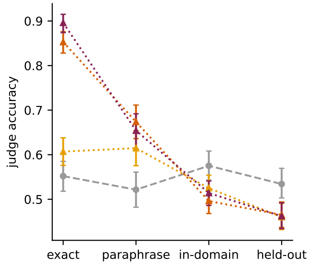
Llama 3.1 8B
