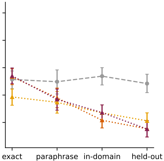
Qwen3-8B
