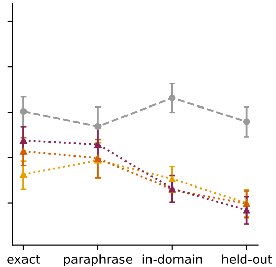
Gemma 4 E4B
