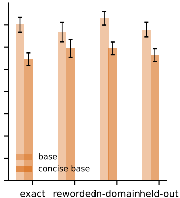
Gemma 4 E4B
