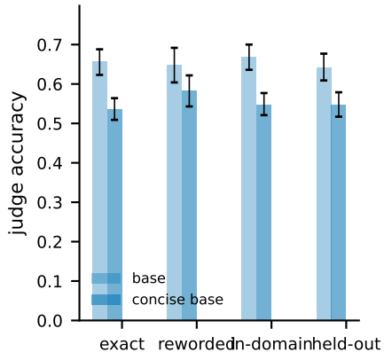
Qwen3-8B
