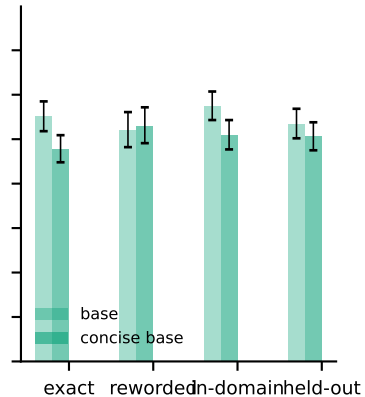
Llama 3.1 8B
