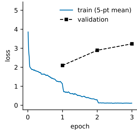
Qwen3-8B
