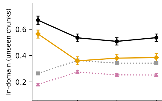
Qwen3-8B
