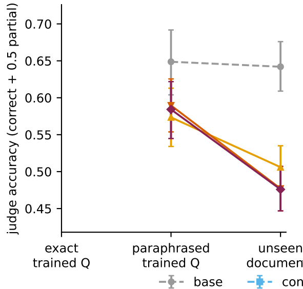
Qwen3-8B
