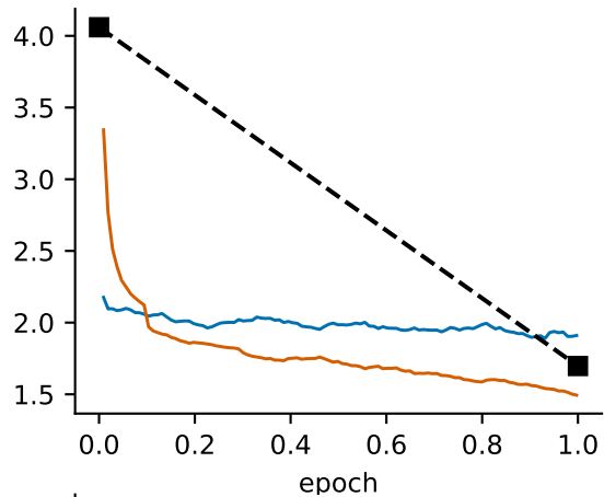
Qwen3-8B
