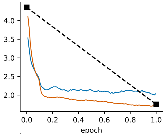
Gemma 4 E4B
