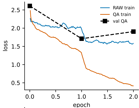
Llama 3.1 8B
