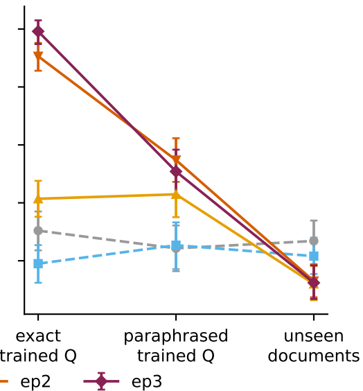
Llama 3.1 8B
