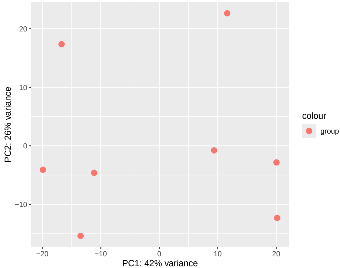
PCA (VST)
