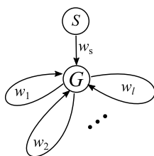
図 10.4.1.7 G(V, E)
