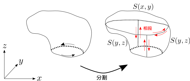
図 8.2.8.1 S の分割
