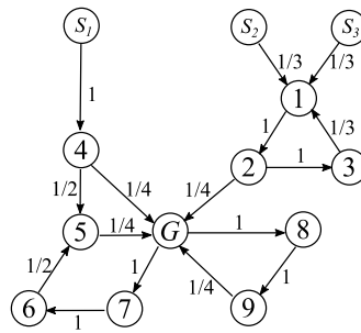
図 8.4.1.1 G(V, E)
