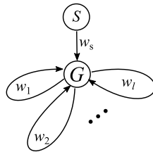
図 8.4.1.8 G(V, E)
