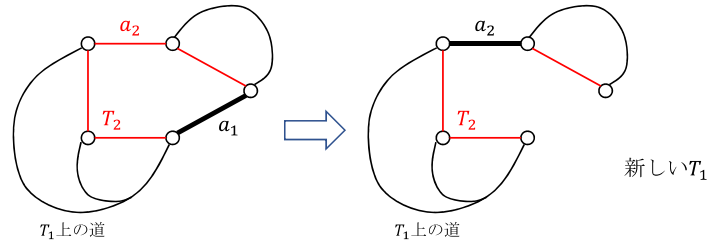
図 8.3.1.2 辺を取り替えて新しい T_1 を作る
