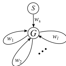
図 8.4.1.7 G(V, E)
