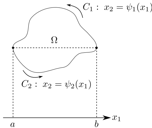
図 4.21.3.1 積分領域
