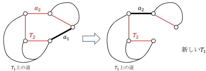
図 10.3.1.2 辺を取り替えて新しい T_1 を作る
