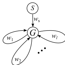
図 9.4.1.7 G(V, E)
