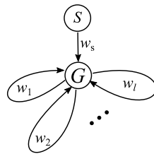
図 VIII.4.7 G(V, E)
