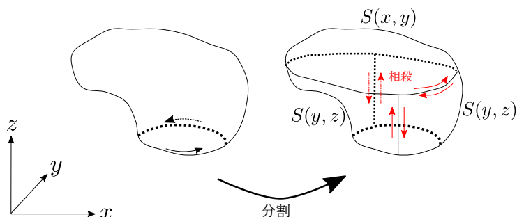
図 VII.1.1 S の分割
